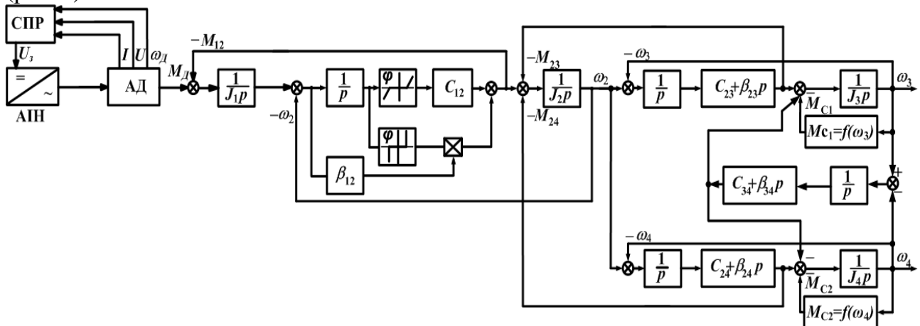
Рис.3 Структурна схема електромеханічної системи з електроприводом змінного струму: U_3 - напруга завдання; I , U , \omega_{д} - поточні значення струму, напруги та швидкості двигуна.
