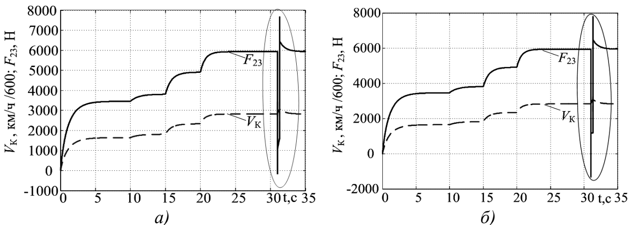
Рис.5 Динамічні процеси в чотирьохмасовій моделі при переміщенні робочої точки по зростаючій ділянці АВ (а) і при переміщенні з ділянки АВ на DC (б): F_{23} - пружна сила в півосі колісної пари; V_k лінійна швидкість колісної пари
