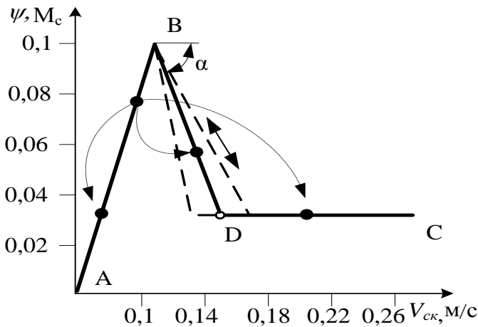
Рис. 4. Характеристика зчеплення, що використовувався для моделювання: \alpha - кут нахилу падаючої ділянки
