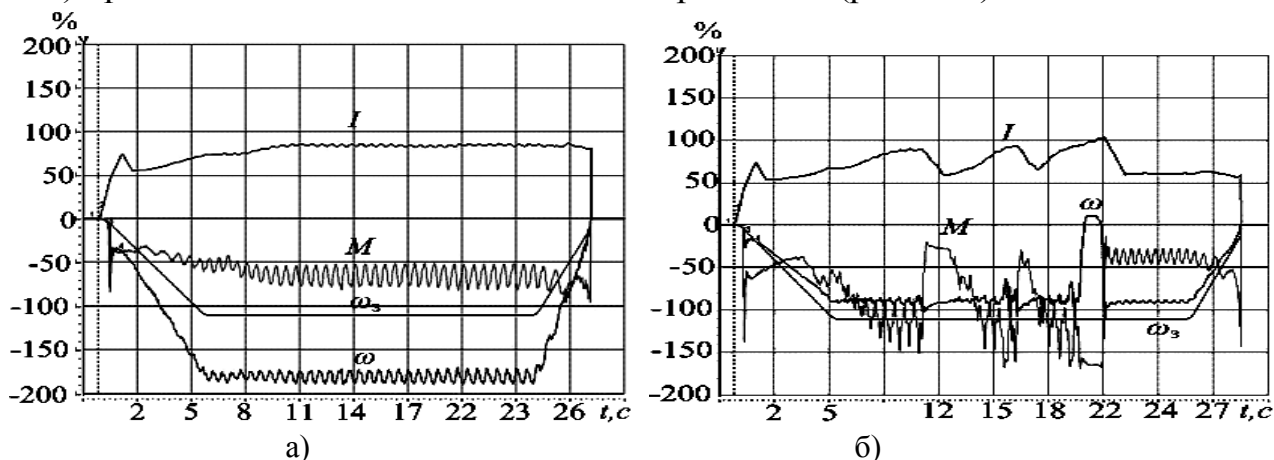
Рис. 12 Осцилограми нестационарного режиму роботи експериментального стенду: I , M , \omega - поточні значення струму моменту і швидкості двигуна; \omega_3 - значення завдання швидкості після задатчика інтенсивності.
