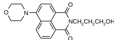
4-Морфоліно-N-(β-гідрокси- пропіл)-нафталімід
