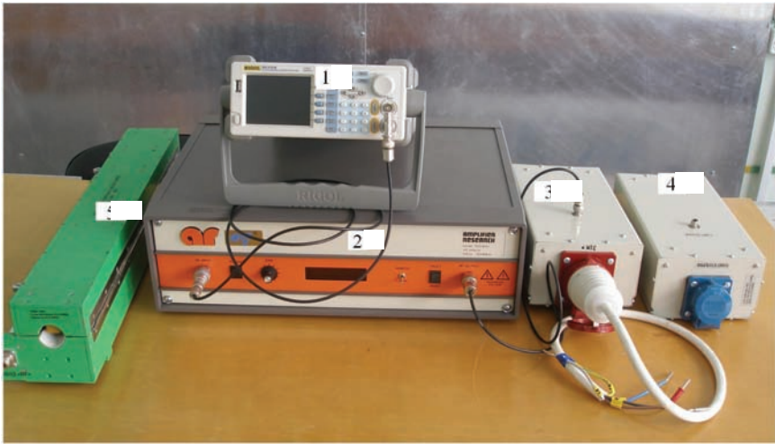
Рисунок 1 – Общий вид установки У-КП-80:
