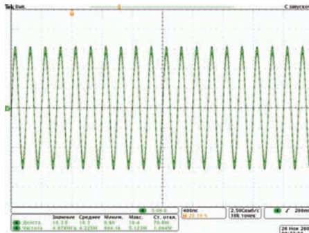
Рисунок 3 – Типовая осциллограмма не модулированного выходного напряжения U_{эфф} = 10 В на частоте 10 МГц (без УСР)
