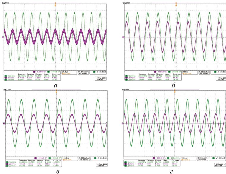
Рисунок 9 – Типовые осциллограммы калибровочного тока (большая синусоида) и напряжение на выходе ТС-А (меньшая синусоида) на различных калибровочных частотах: а – F = 60 \text{ кГц} ; б – F = 10 \text{ МГц} ; в – F = 20 \text{ МГц} ; г – F = 100 \text{ МГц}
