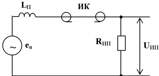
Рисунок 6 – Схема замещения ТС-А
