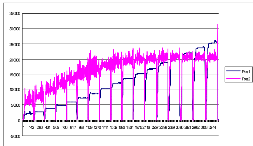
Рис.2 Относительная неопределенность
