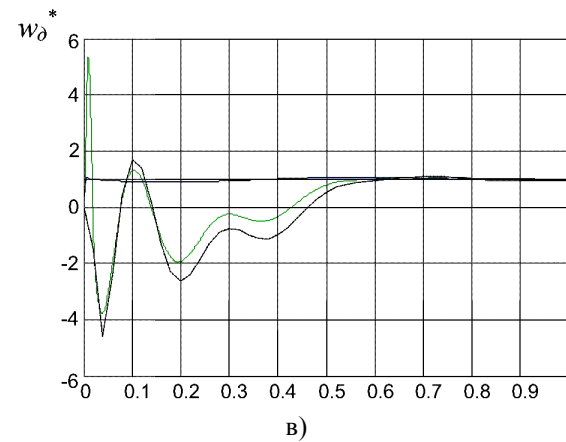
Рис. 1. Переходные процессы в робастной системе управления по задающему воздействию
