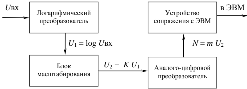
Рис.1. Структурная схема преобразователя сигнала ЯМР
