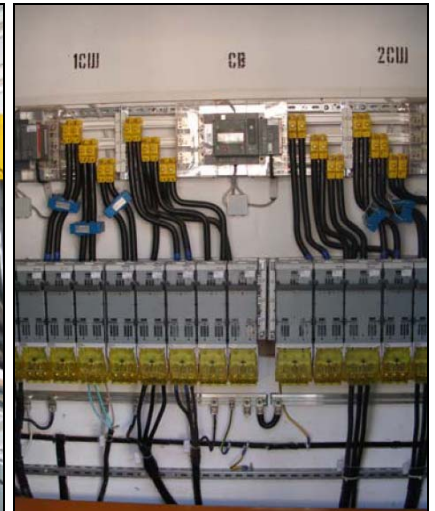
РП-0,4 ЗАВОДУ СКЛОТАРИ (м. Буча, Київська обл.)
