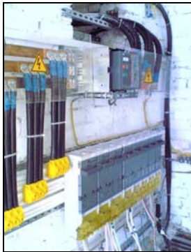
РП-0,4 ТРАНСФОРМАТОРНОЇ ПІДСТАНЦІЇ ТП-468 (м. Житомир)
