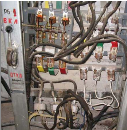
РП-0,4 ТРАНСФОРМАТОРНОЇ ПІДСТАНЦІЇ ТП-468 (м. Житомир)
