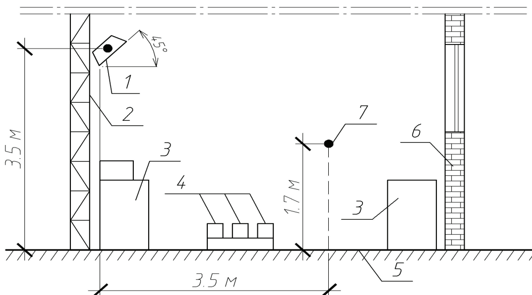
Рис. 1. Схема расположения инфракрасного трубчатого нагревателя и различного оборудования на участке проведения экспериментальных работ (поперечный разрез): 1 – инфракрасный нагреватель; 2 – колонна; 3 – металлообрабатывающее оборудование; 4 – местный склад готовых обработанных деталей; 5 – пол; 6 – кирпичная наружная стена цеха; 7 – линия, вдоль которой производились замеры параметров
