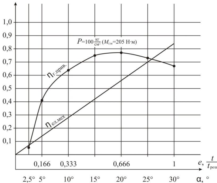
Рис. 1 Залежності ККД гідростатичного \eta і електромеханічного \eta_{\text{ел.мех.}} приводів від від кута повороту люльки насоса \alpha , відносної продуктивності e і відносної швидкості розгону t/t_{\text{розг}}
