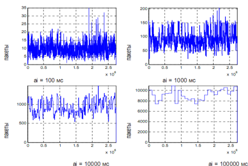
Рис. 1. Реализации трафика
