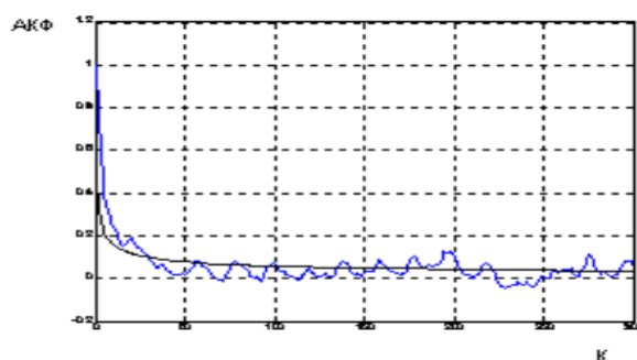
Рис. 2. Автокорреляционная функция
