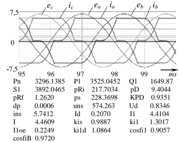
Рис. 7. Диаграммы напряжений и токов источника, распечатка расчетных величин выпрямителя
