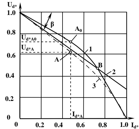
Рис. 2. Внешние характеристики трехфазного выпрямителя
