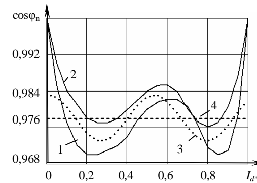
Рис. 6. Зависимости \cos\varphi_n(I_{d^*}) .
